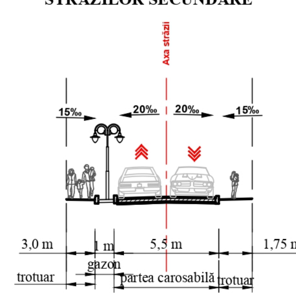
PROFIL TRANSVERSAL (Secțiunea 3:3 - 3:3) EXEMPLU DE DEZVOLTARE AL STRĂZILOR SECUNDARE
